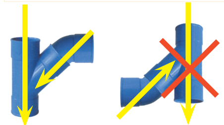
Kein Kleber in die Innenseite
