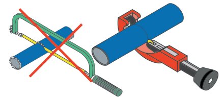
Gerade Ablängen und Entgraten
