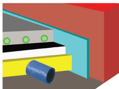
Verlegung am Rohboden
