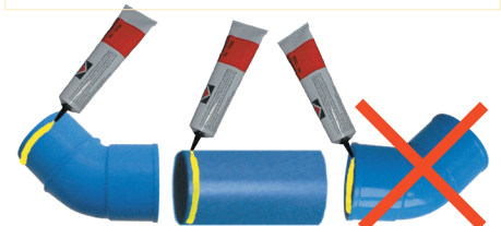
Kein Kleber in die Innenseite
